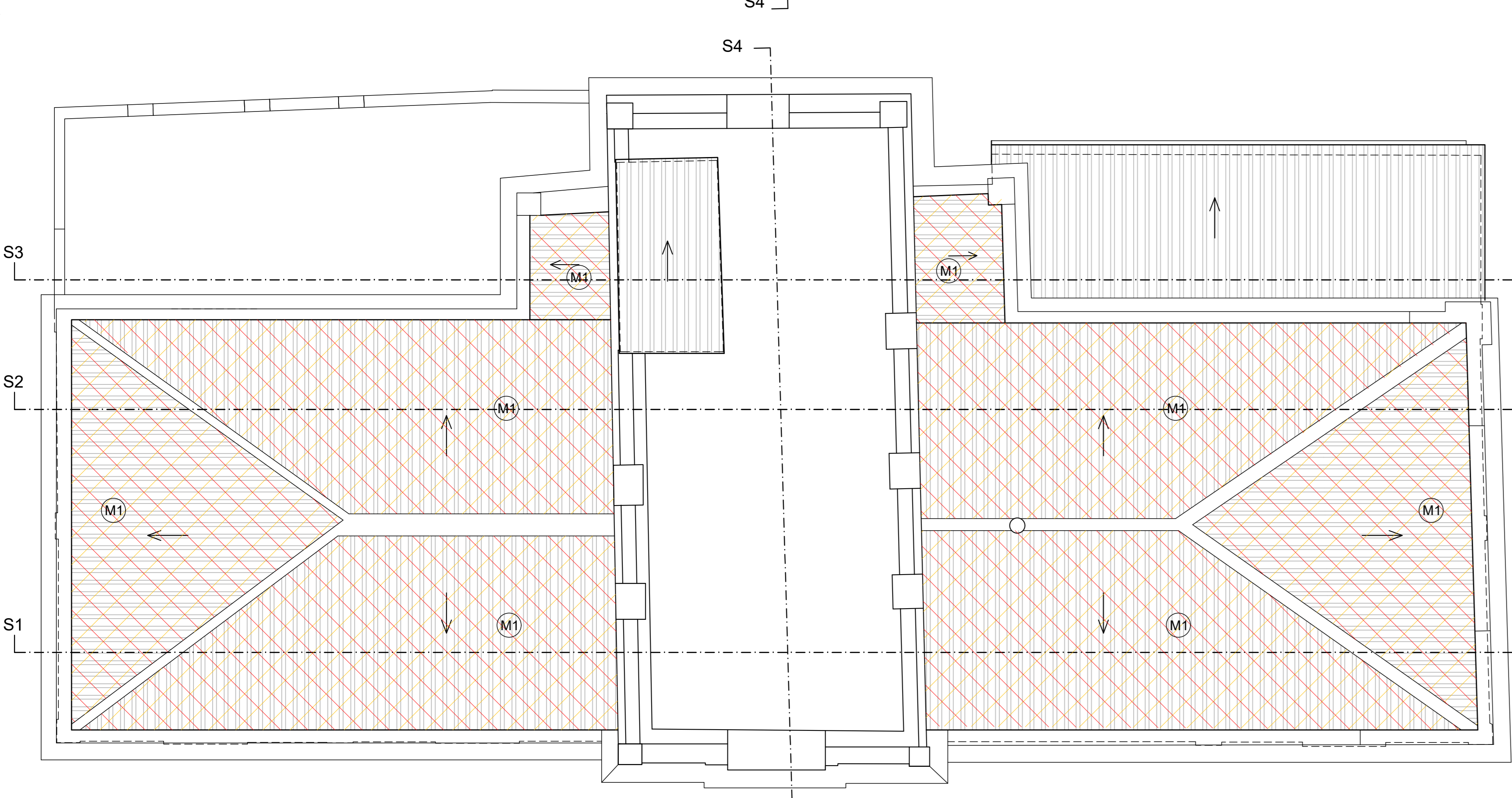
PIANTA COPERTURA
